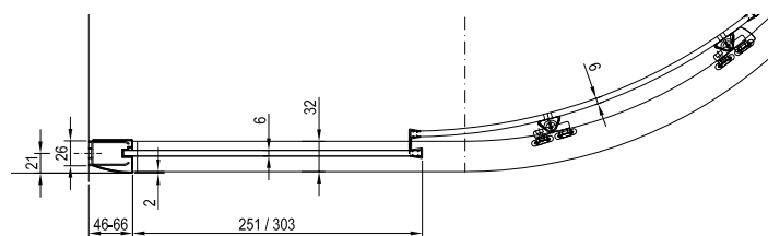
Dušas kabīnes BLCP4 ir BLCP4 Sabina rasējums
