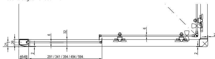
Dušas kabīnes BLRV2 ir BLRV2K rasējums
